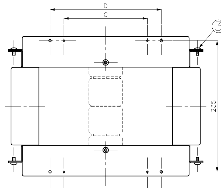
底面図 (F / )
